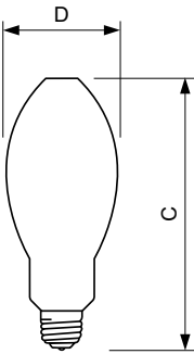
MHC 150W/940 E26 BD17 CO U
