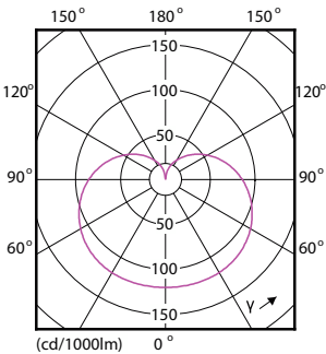
Light Distribution Diagram - 14A19/COR/940/FR/P/E26/DIM/T20 6/1CT
